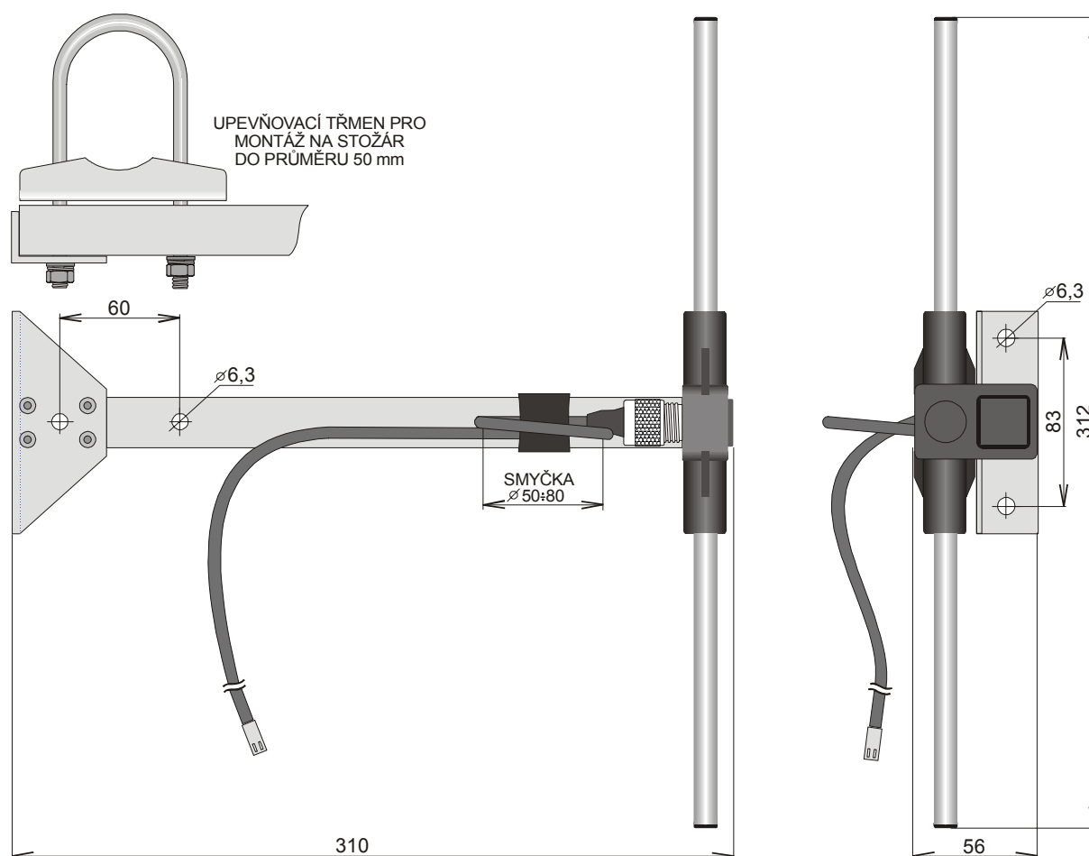
mechanické rozměry antény AN-03
